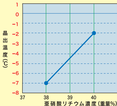
亜硝酸リチウムと濃度と晶出温度との関係
