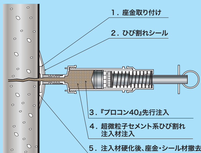
超微粒子セメント系注入材本注入の状況
